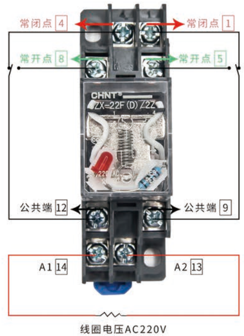
(24V继电器脚位图)
